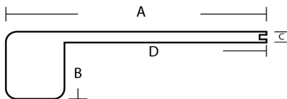
Square Edge Flush Stairnose - 48"(1219mm)
