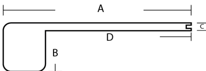
Square Edge Flush Stairnose - 72"(1829mm)
